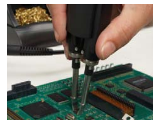
Sistema MX-5041 con Pinza Termica MX-PTZ
